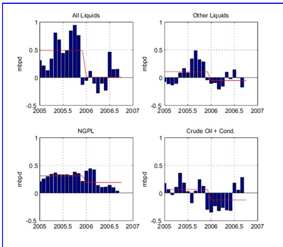
Fig 2.- Révisions cumulées sur les estimations mensuelles de production de l'EIA. Cliquez sur l'image pour agrandir.
