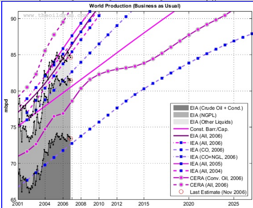
Fig 5.- Prévisions sans maximum de production visible. Cliquez sur l'image pour agrandir.
