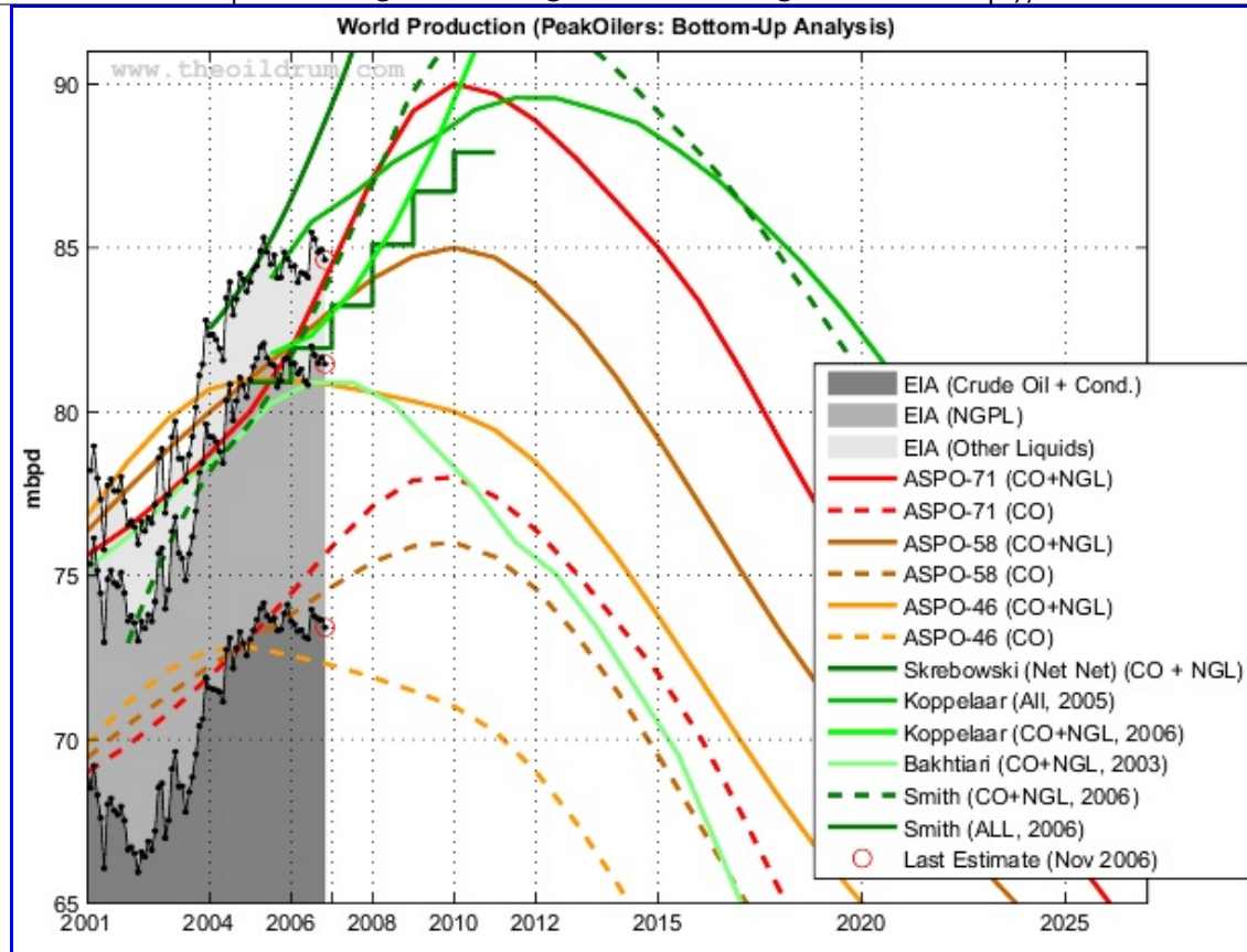
Fig 6.- Prvisions basées sur une analyse détaillée de la production (du bas vers le haut). Cliquez sur l'image pour agrandir.
