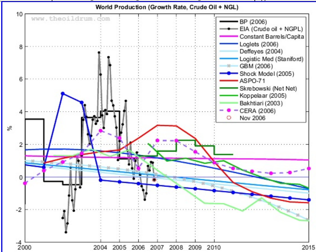
Fig 8.- Croissance de la production entre le mois courant et le même mois de l'année précédente. Cliquez sur l'image pour agrandir.
