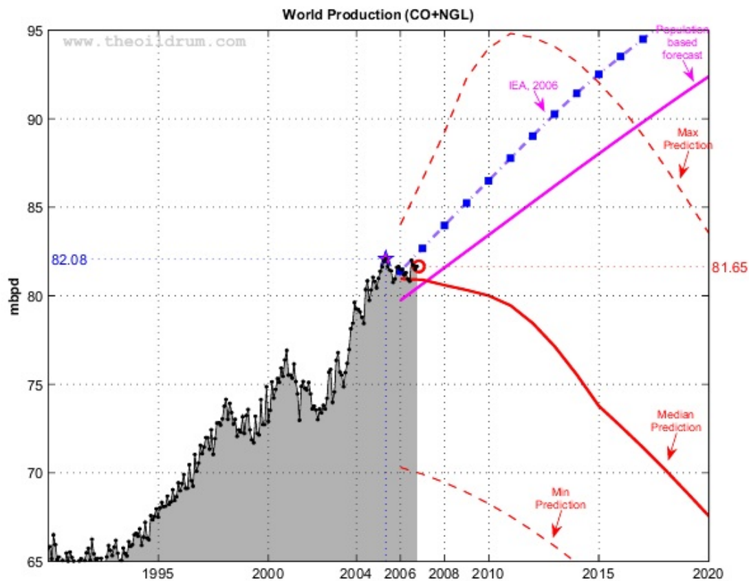
Fig 1.- Production mondiale mensuelle (EIA mensuelle) pour pétrole brut + NGL. Le modèle médian est calculé à partir de la médiane des 9 modèles qui prévoient un pic avant 2020 (Bakhtiari, Smith, Staniford, Loglets, Shock model, GBM, ASPO-[70,58,45]). Cliquez pour agrandir.
