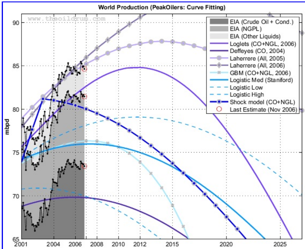
Fig 7.- Prévisions basées sur des approches à base de courbes. Cliquez sur l'image pour agrandir.
