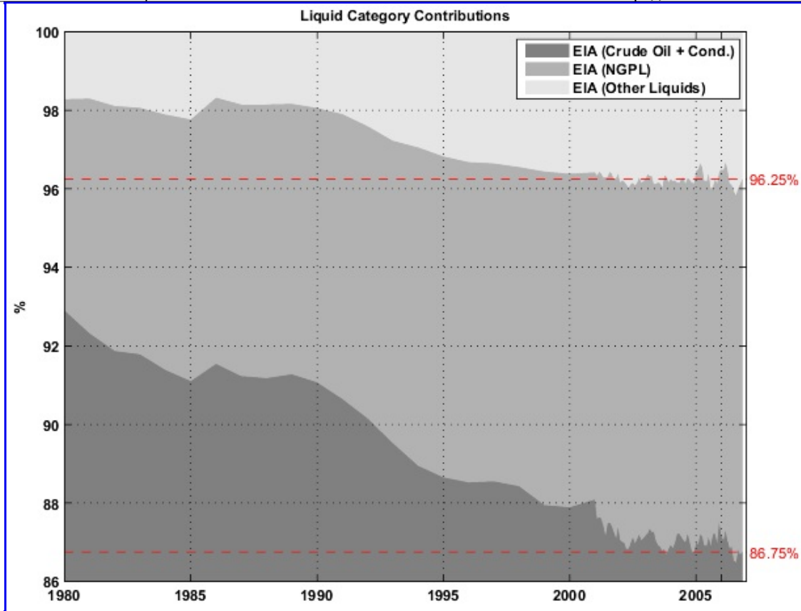
Fig 3.- Contribution de chaque catégorie à la production totale. Cliquez sur l'image pour agrandir.
